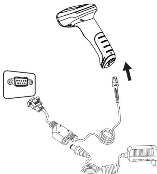
Рисунок 7. Подключение АТОЛ SB5100 с помощью RS-232 - кабеля
