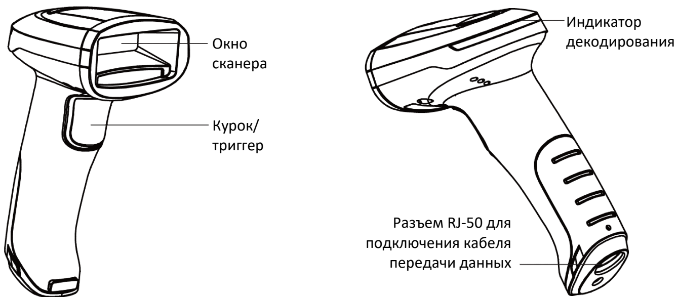
Рисунок 1. Внешний вид сканера АТОЛ SB5100 (вид спереди/слева и вид сзади/снизу/слева)
