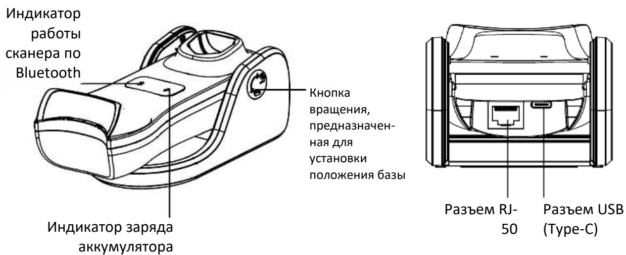
Рисунок 4. Внешний вид базы сканера АТОЛ SB5100 BL
